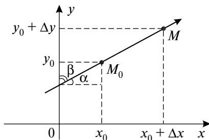
Рис. 26.1. Направление \vec{l} = (\cos \alpha, \cos \beta) .
