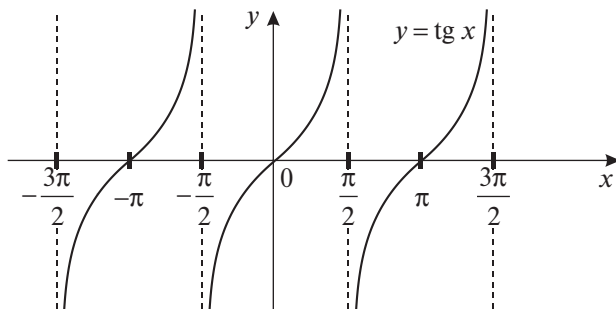
Рис. 13.9. График функции y = \operatorname{tg} x
