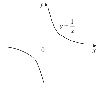
Рис. 13.3. График степенной функции y = x^a при a = -1
