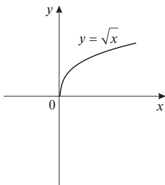
Рис. 13.4. График степенной функции y = x^a при a = \frac{1}{2}
