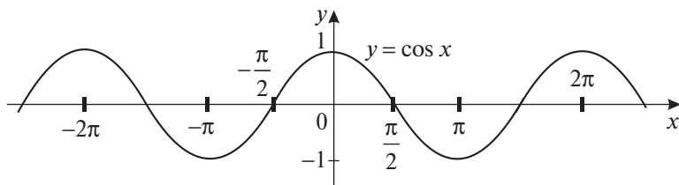
Рис. 13.8. График функции y = \cos x
