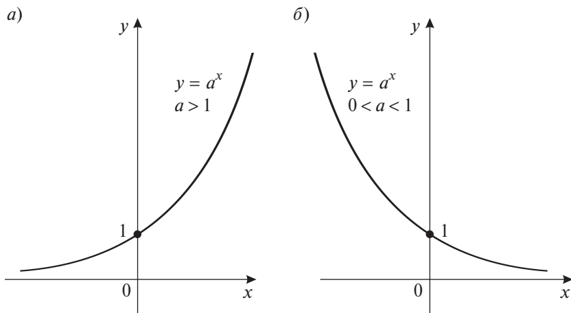
Рис. 13.5. График показательной функции y = a^x при a > 1 (а) и при 0 < a < 1 (б)
