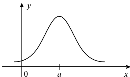
Рис. 19.3. Нормальная кривая
