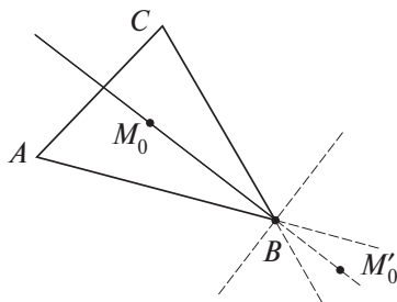
Рис. 7.4. Биссектриса внутреннего угла треугольника ABC
