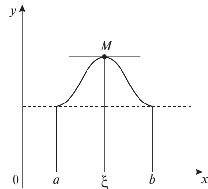
Рис. 17.2. Геометрический смысл теоремы Ролля
