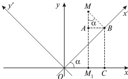
Рис. 8.6. Поворот системы координат
