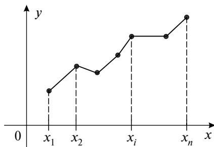
Рис. 27.1. Экспериментальная кривая
