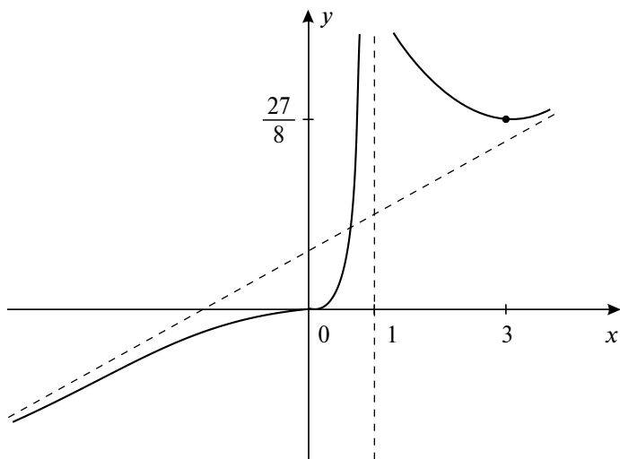
Рис. 19.2. График функции y = \frac{x^3}{2(x-1)^2}
