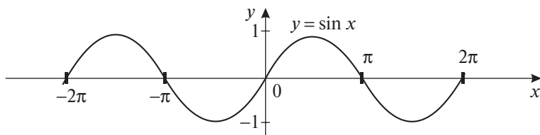
Рис. 13.7. График функции y = \sin x
