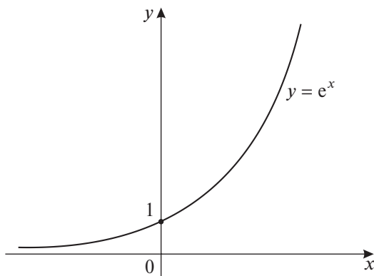
Рис. 14.3. Экспонента
