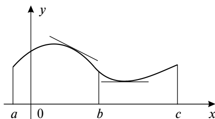
Рис. 19.1. Направление выпуклости графика
