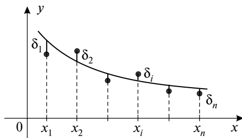
Рис. 27.3. Иллюстрация метода наименьших квадратов
