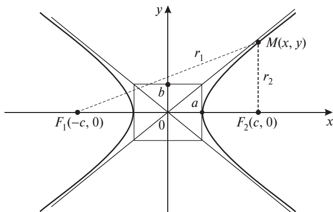
Рис. 8.3. Гипербола \frac{x^2}{a^2} - \frac{y^2}{b^2} = 1
