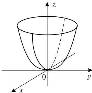
Рис. 25.2. График функции z = x^2 + y^2
