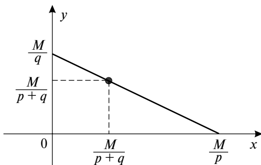
Рис. 28.2. Максимум функции полезности
