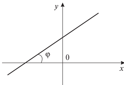
Рис. 7.2. Прямая с угловым коэффициентом k = \operatorname{tg} \varphi
