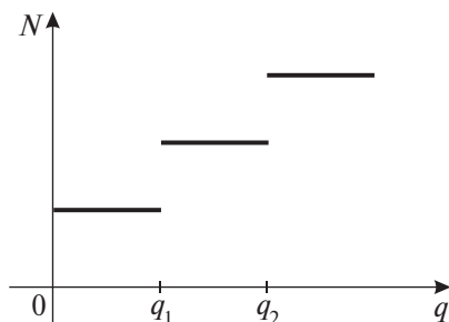
Рис. 15.1. Налоговая ставка
