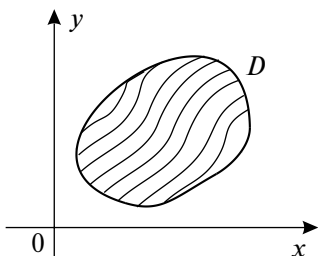
Рис. 29.1. Интегральные кривые
