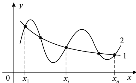
Рис. 27.2. Определение общего вида зависимости y = f(x)
