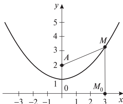
Рис. 7.1. Парабола y = \frac{x^2}{4} + 1
