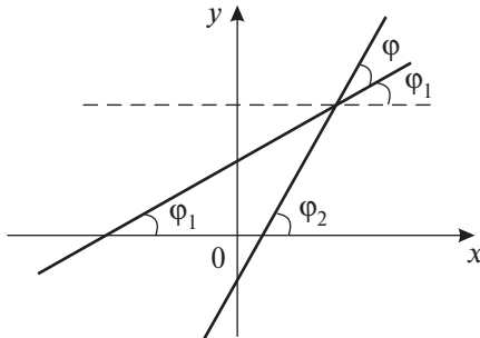
Рис. 7.3. Угол \varphi между прямыми
