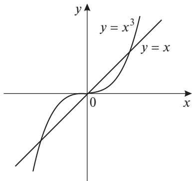
Рис. 13.2. График степенной функции y = x^a при a = 1 и a = 3
