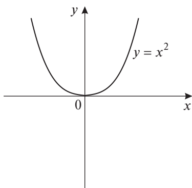
Рис. 13.1. График степенной функции y = x^a при a = 2
