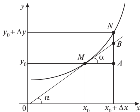
Рис. 16.2. Геометрический смысл дифференциала
