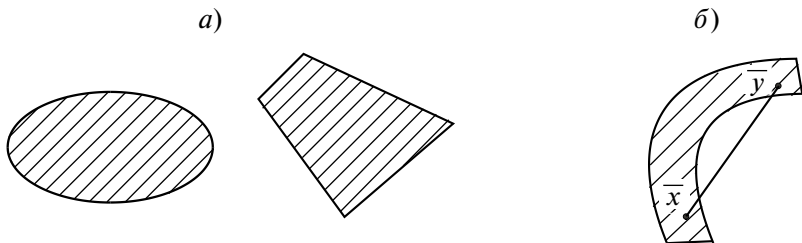
Рис. 28.1. Множества: выпуклые (а) и невыпуклое (б)
