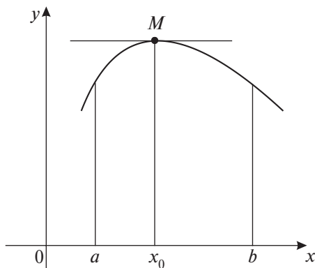
Рис. 17.1. Геометрический смысл теоремы Ферма
