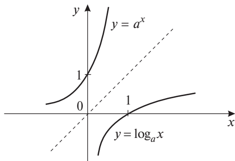
Рис. 13.11. Графики взаимно обратных функций y = a^x и y = \log_a x
