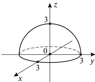
Рис. 25.1. График функции z = \sqrt{9 - x^2 - y^2}
