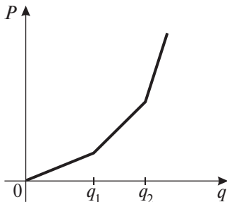
Рис. 15.2. Подоходный налог
