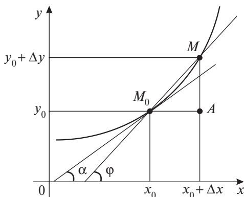
Рис. 16.1. Геометрический смысл производной
