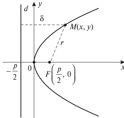
Рис. 8.4. Парабола y^2 = 2px
