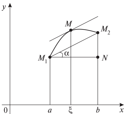
Рис. 17.3. Геометрический смысл теоремы Лагранжа
