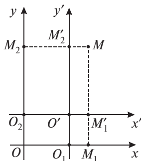
Рис. 8.5. Параллельный перенос системы координат
