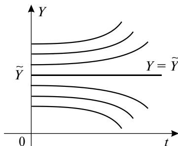
Рис. 29.2. Интегральные кривые уравнения (29.20)
