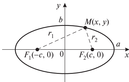
Рис. 8.2. Эллипс \frac{x^2}{a^2} + \frac{y^2}{b^2} = 1
