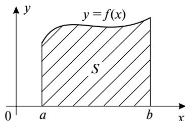
Рис. 22.2. Геометрический смысл определенного интеграла
