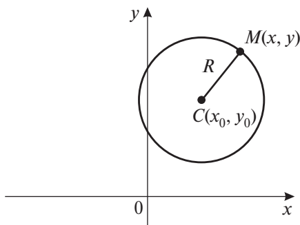
Рис. 8.1. Окружность с центром в точке C и радиусом R = CM
