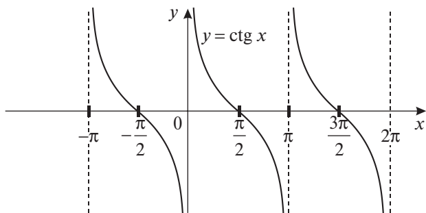
Рис. 13.10. График функции y = \operatorname{ctg} x
