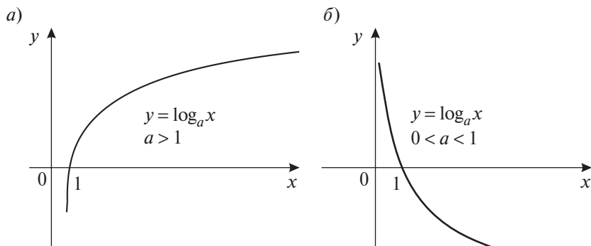
Рис. 13.6. График логарифмической функции y = \log_a x при a > 1 (а) и при 0 < a < 1 (б)
